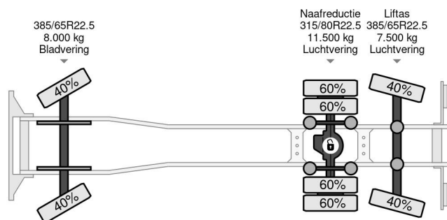
Mercedes-Benz Arocs 2546 | 6X2*4 | JUNJIN 25 METER | R...
