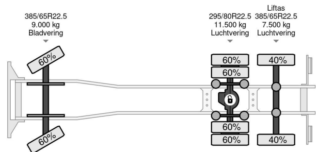
Mercedes-Benz Actros 2653 6X2 | RETARDER | HYVA HOOK...
