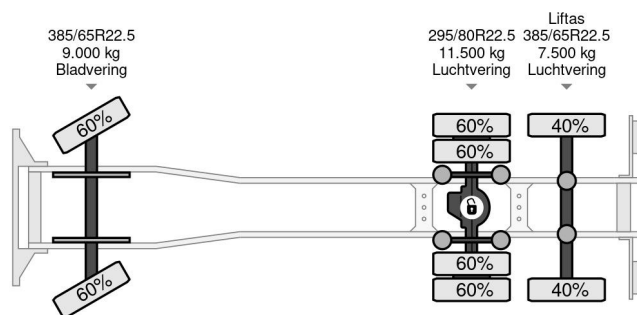
Mercedes-Benz Actros 2653 6X2 | RETARDER | HYVA HOO...
